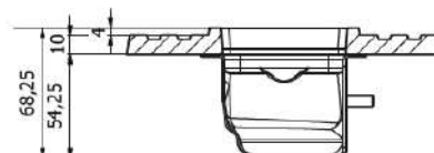
A-A ( 1/2 )
